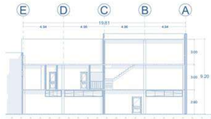
CORTE TRANSVERSAL (OFICINAS)
