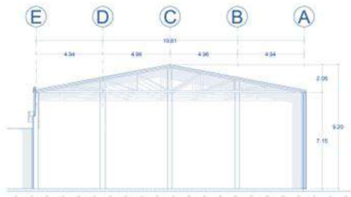
CORTE TRANSVERSAL (NAVE)
