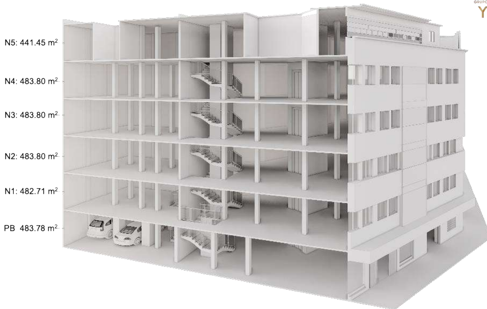
CORTE ESQUEMÁTICO
