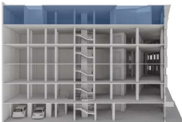
CORTE ESQUEMÁTICO
